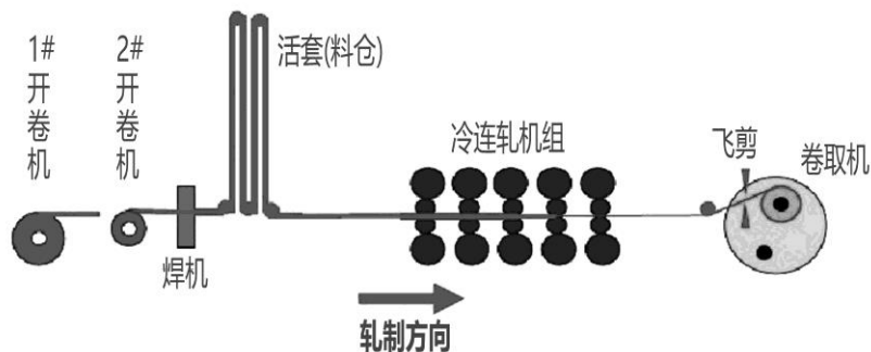
冷轧板轧制工艺流程图
