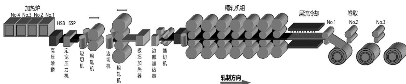
热轧板轧制工艺与减速机布置图
