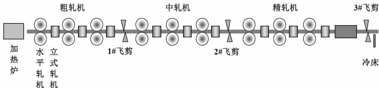
棒线材轧制工艺与减速机布置图
