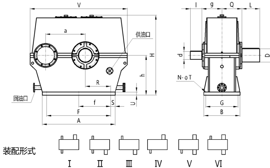
MBY 系列减速机外形尺寸
