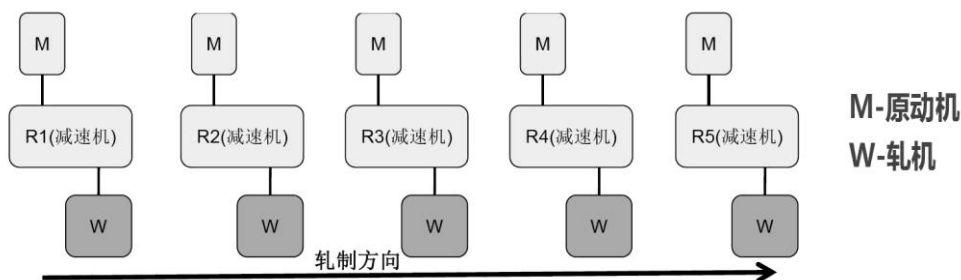
冷轧板轧机专用减速机布置图
