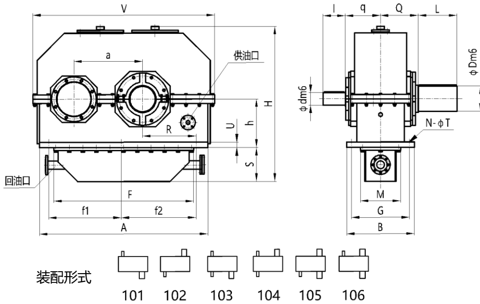
JDX 系列减速机外形尺寸
